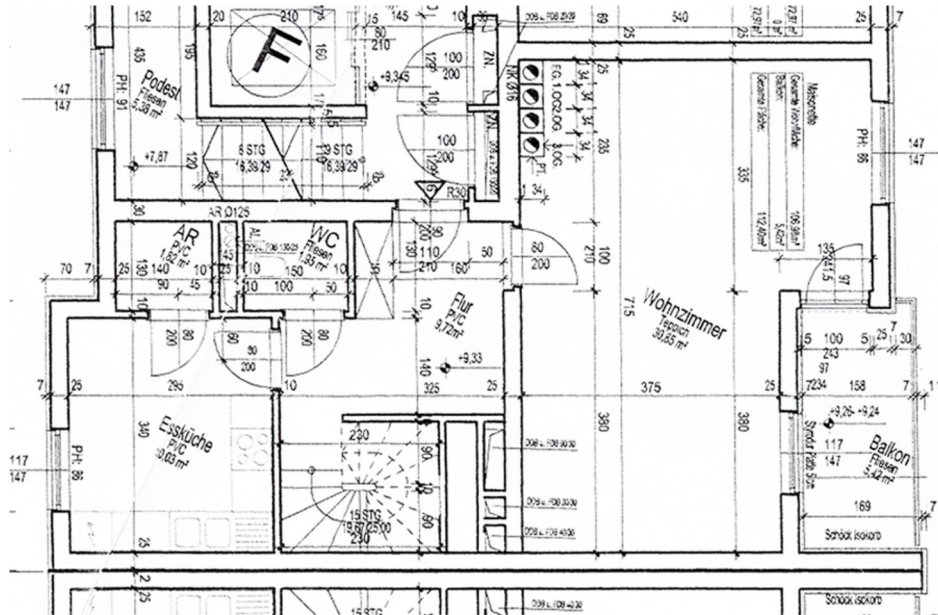
3. Obergeschoss
